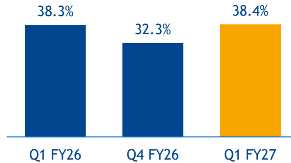
PCR
